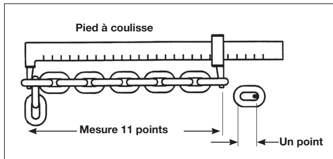
Figure 7 - Inspection de la chaîne
