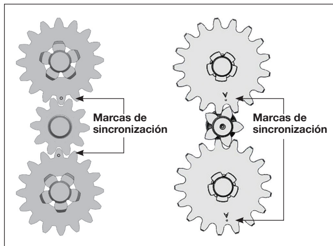
Figura 10 - Sincronización de engranajes (0,75 y 1,5 toneladas)
