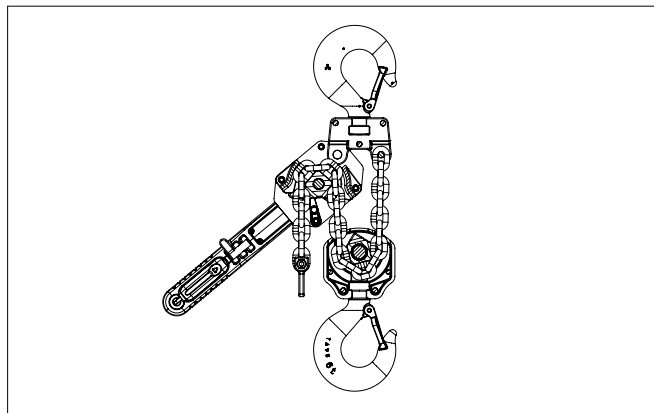
Instalación de la cadena de doble caída (6 Tonne)
