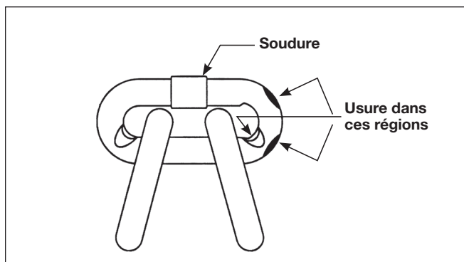
Figure 6 - Inspection de la chaîne
