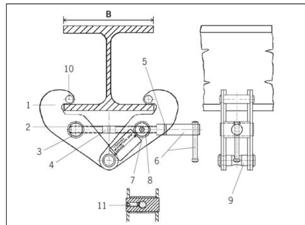
FIGURE 2: PINCE À POUTRE 10 TONNE
