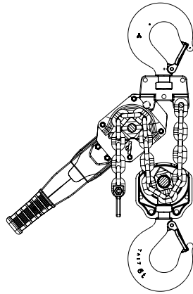
Installation de la chaîne à passage unique (6 tonnes)
